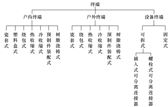
图 1 终端系列型谱
